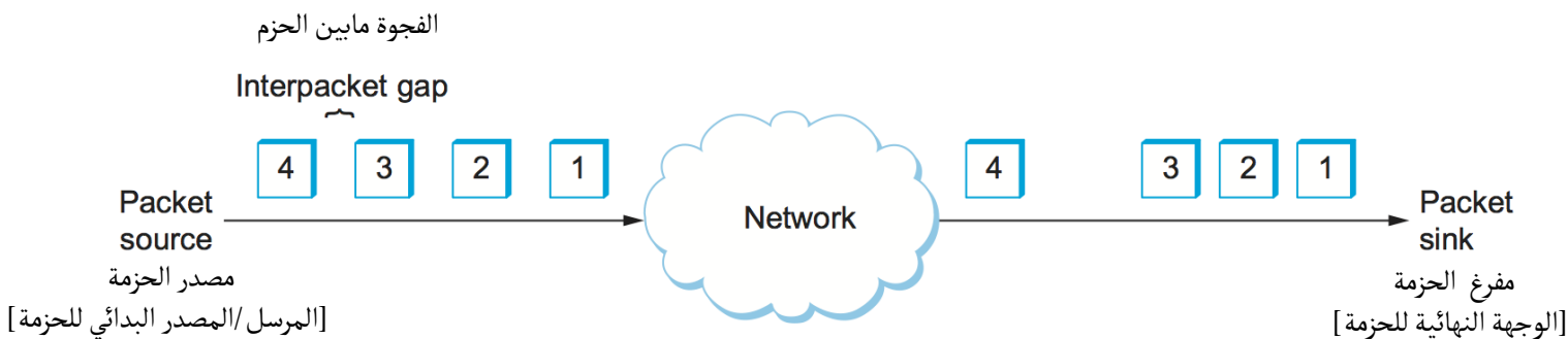
الشكل 5: تذبذب في التأخير delay jitter ناتج عن الشبكة induced by the network
